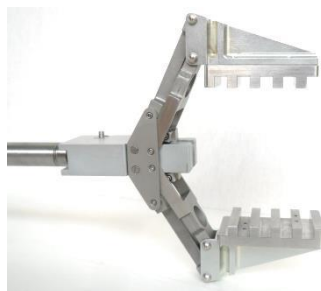
Mors parallèles spéciaux pour lever des sacs Special parallel jaws for lifting bags
